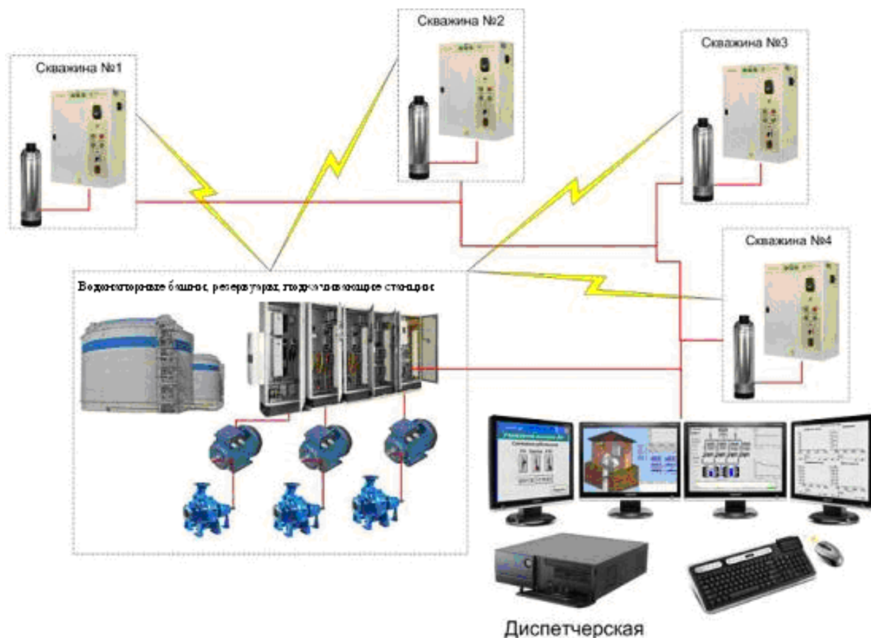
Рисунок 21 – Схема автоматизации, диспетчеризации и управления
