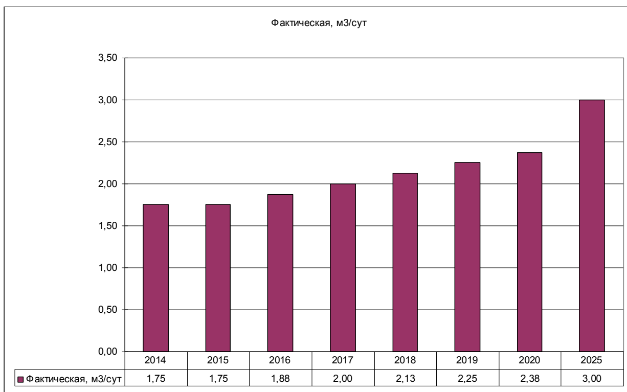
Рисунок 19 – Прогноз перспективного среднесуточного потребления воды д. Бегешка
