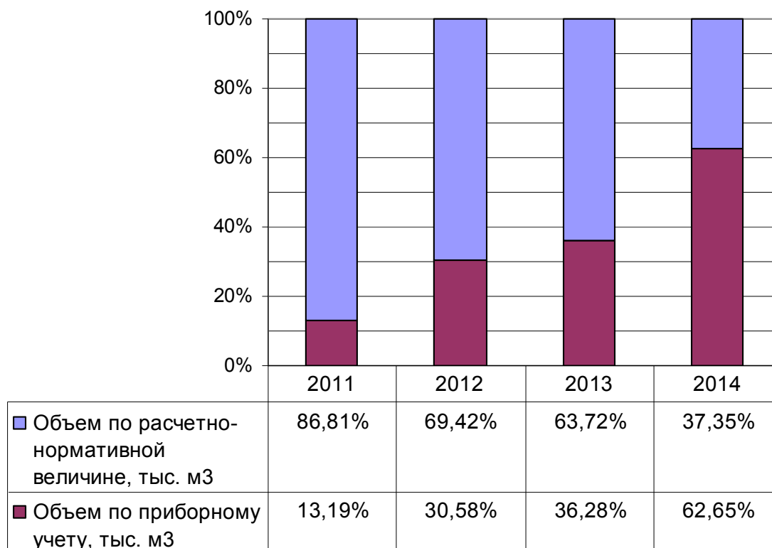
Рисунок 14 – Долевая диаграмма потребляемой воды по приборному учету и расчетно-нормативной величине за период 2011-2014 гг.
