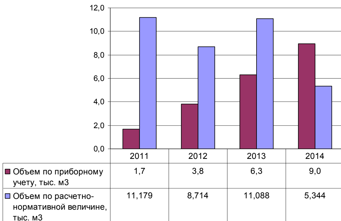
Рисунок 13 – Динамика изменения объемов потребления воды по фактическим и расчетным данным за период с 2011 по 2014 гг.
