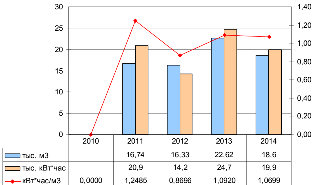
Рисунок 4 – Динамика изменения объемов потребления энергоресурсов скважиной №112 с. Селычка, пер. Санаторный за период с 2010-2014 гг.
