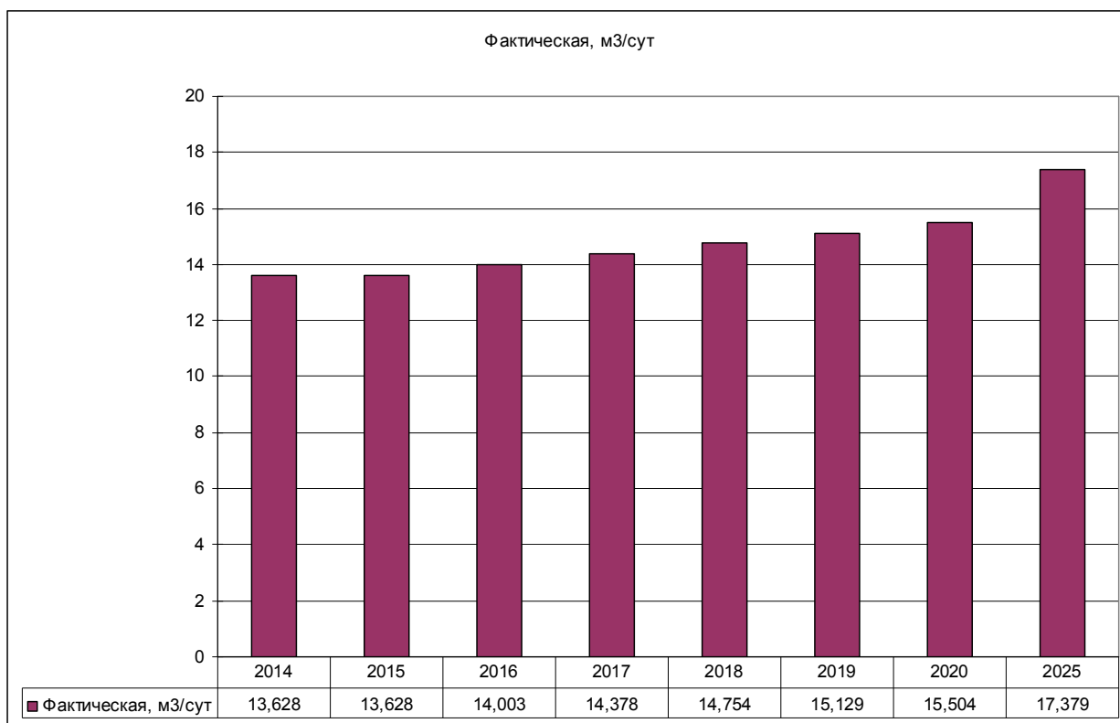
Рисунок 18 – Прогноз перспективного среднесуточного потребления воды д. Солнечный
