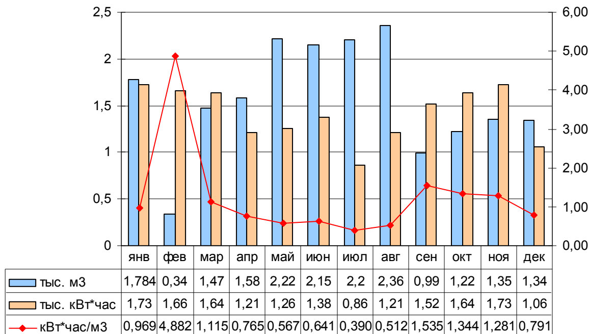
Рисунок 6 – Динамика сезонного изменения объемов потребления электроэнергии скважиной №112 с. Сельчка, пер. Санаторный за 2014г.
