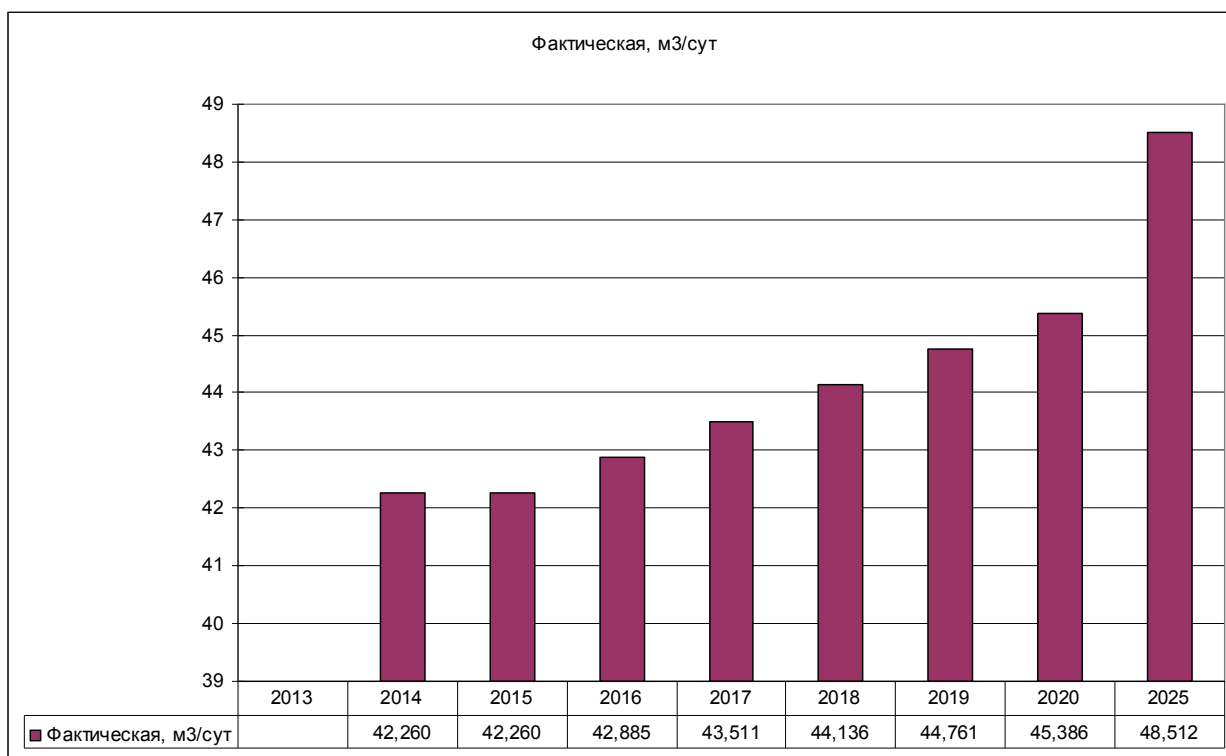
Рисунок 17 – Прогноз перспективного среднесуточного потребления воды с. Канифольный
