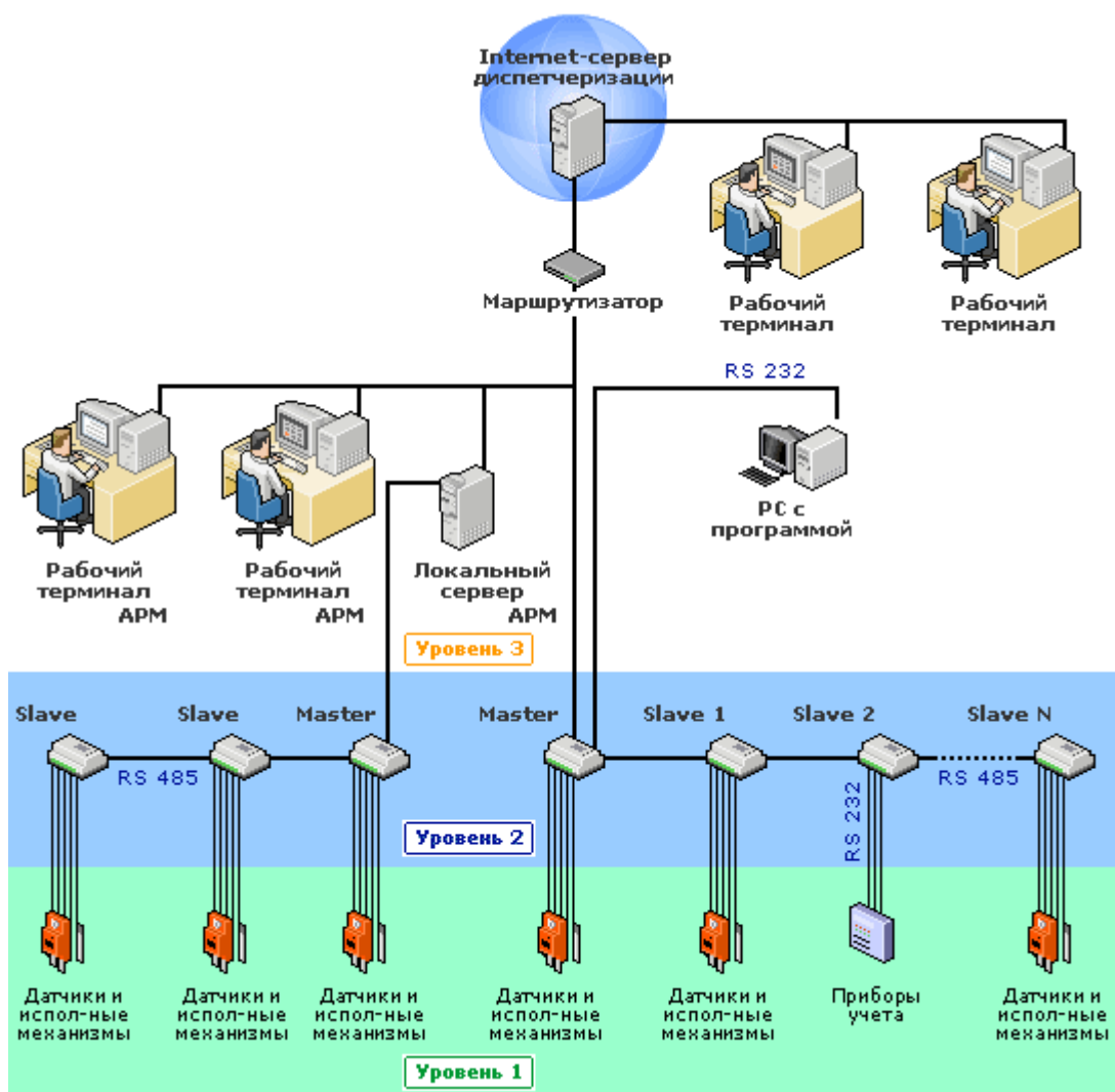
Рисунок 22 – Схема уровней системы АСУ ТП
