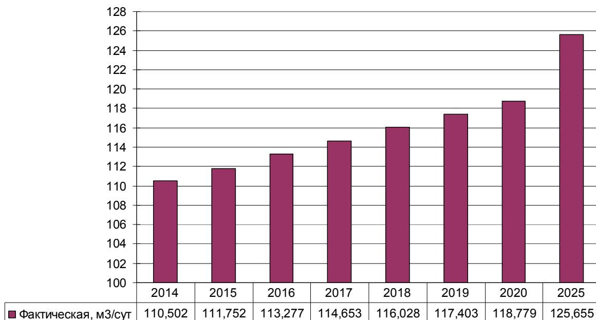
Рисунок 16 – Прогноз перспективного среднесуточного потребления воды с. Сельчка
