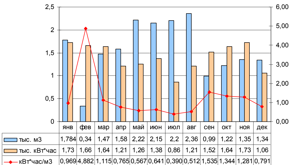
Рисунок 5 – Динамика сезонного изменения объемов потребления электроэнергии скважиной №112 с. Селычка, пер. Санаторный за период с 2010-2014 гг.
