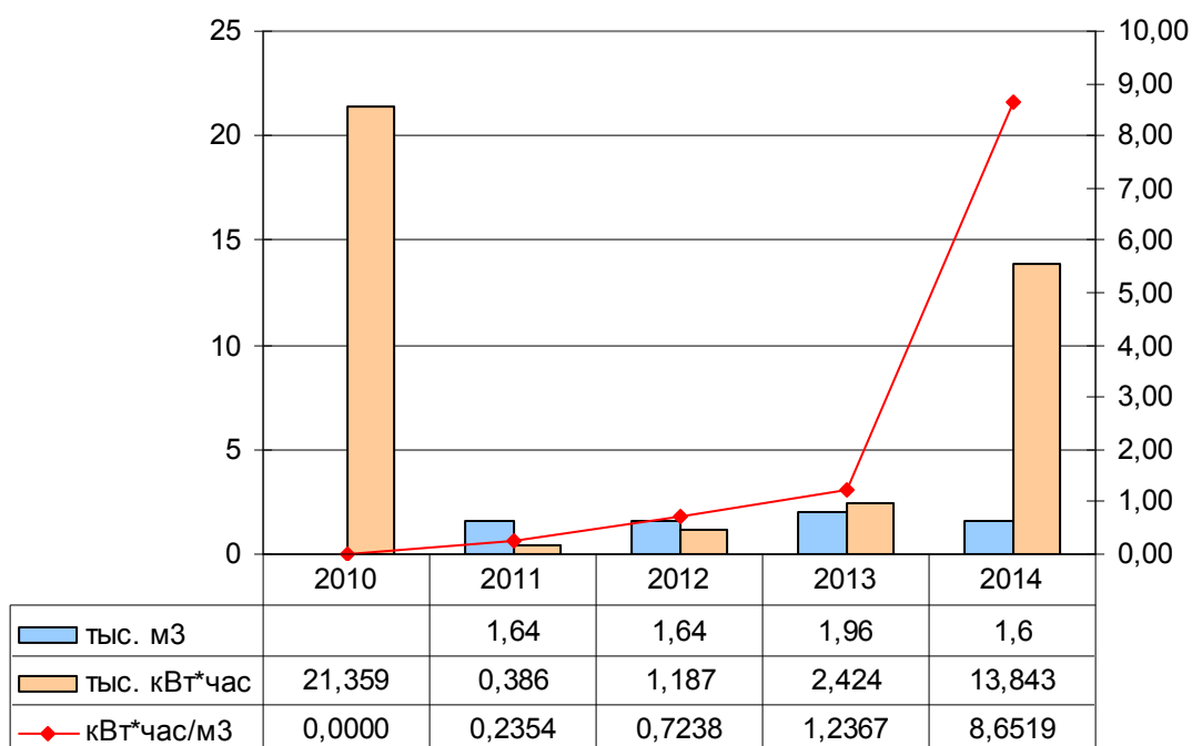
Рисунок 6 – Динамика изменения объемов потребления энергоресурсов скважиной №1423а д.Иж-Забегалово ул.Пушиной 1а за период с 2010-2014 гг.
