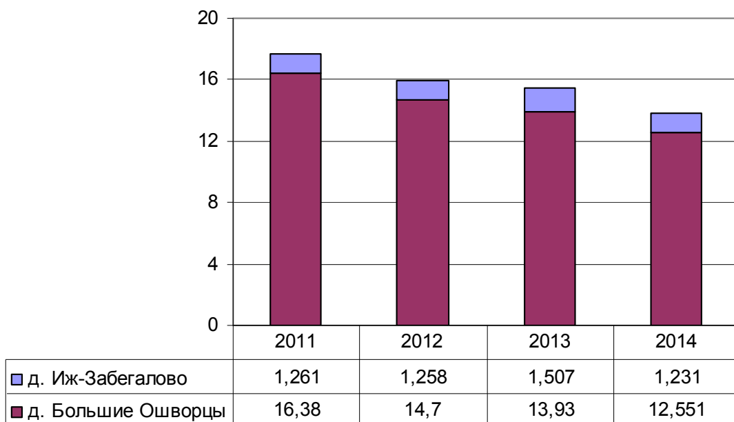
Рисунок 13 – Территориальный баланс подачи воды по технологическим зонам водоснабжения МО «Большеошворцинское»
