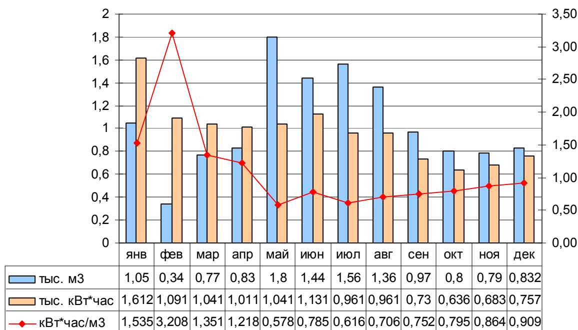
Рисунок 5 – Динамика сезонного изменения объемов потребления электроэнергии скважиной №1423 д.Б.Ошворцы ул.Советская 7а за 2014 г.
