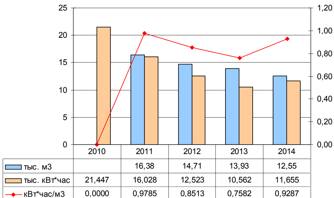
Рисунок 4 – Динамика изменения объемов потребления энергоресурсов скважиной №1423 д.Б.Ошворцы ул.Советская 7а с 2010-2014 гг.
