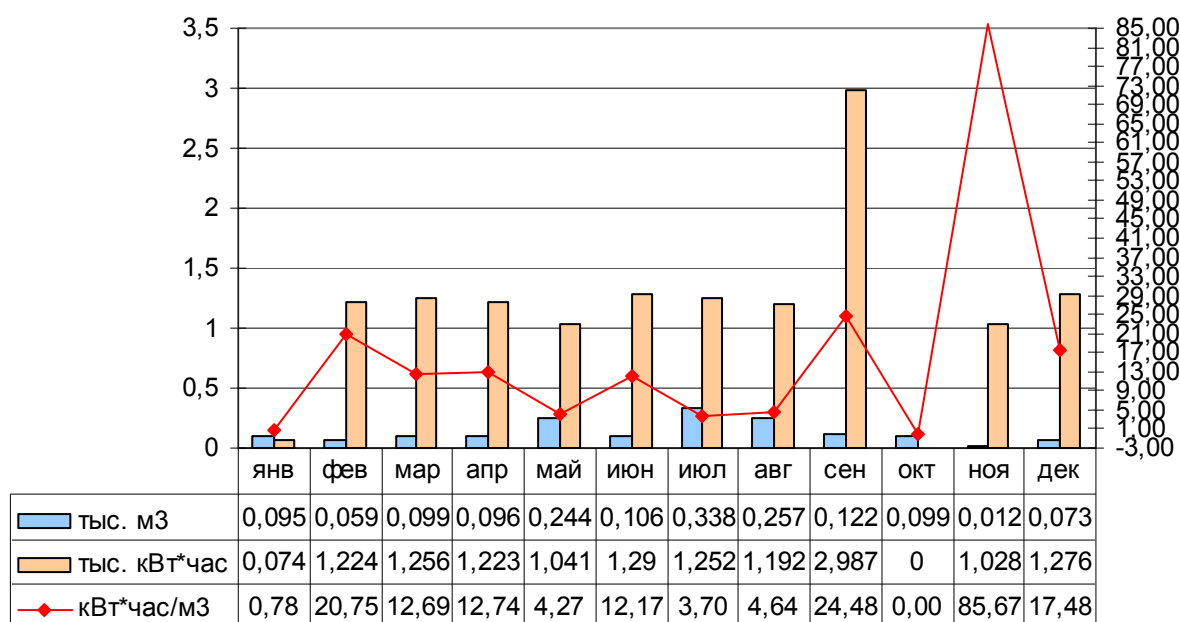
Рисунок 7 – Динамика сезонного изменения объемов потребления электроэнергии скважиной №1423а д.Иж-Забегалово ул.Пушиной 1а за 2014 г..
