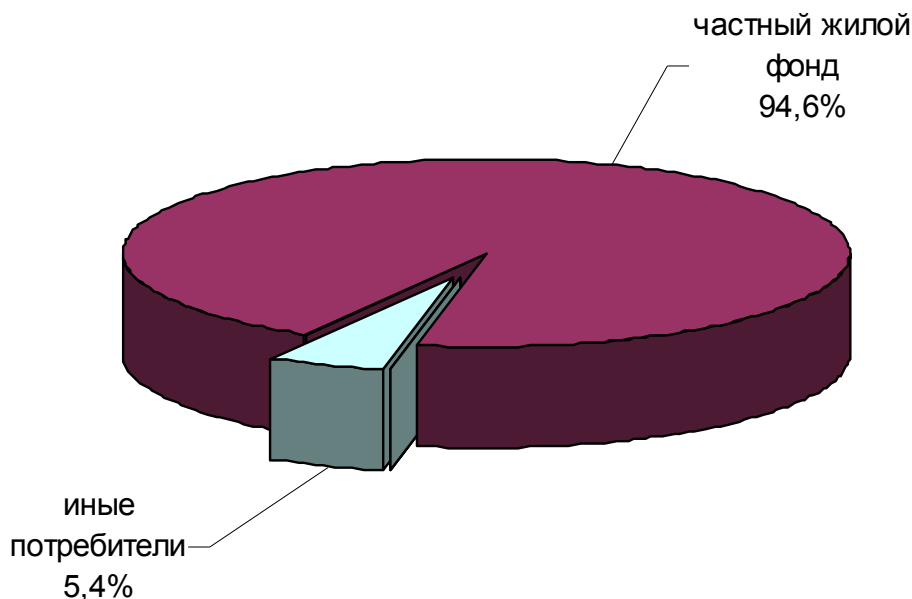
Рисунок 20 – График структурного распределения воды по группам абонентов в 2014 г. д. Иж-Забегалово
